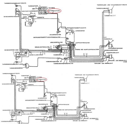
Kabel von Batt. Pluspol zu Startfußschalter
